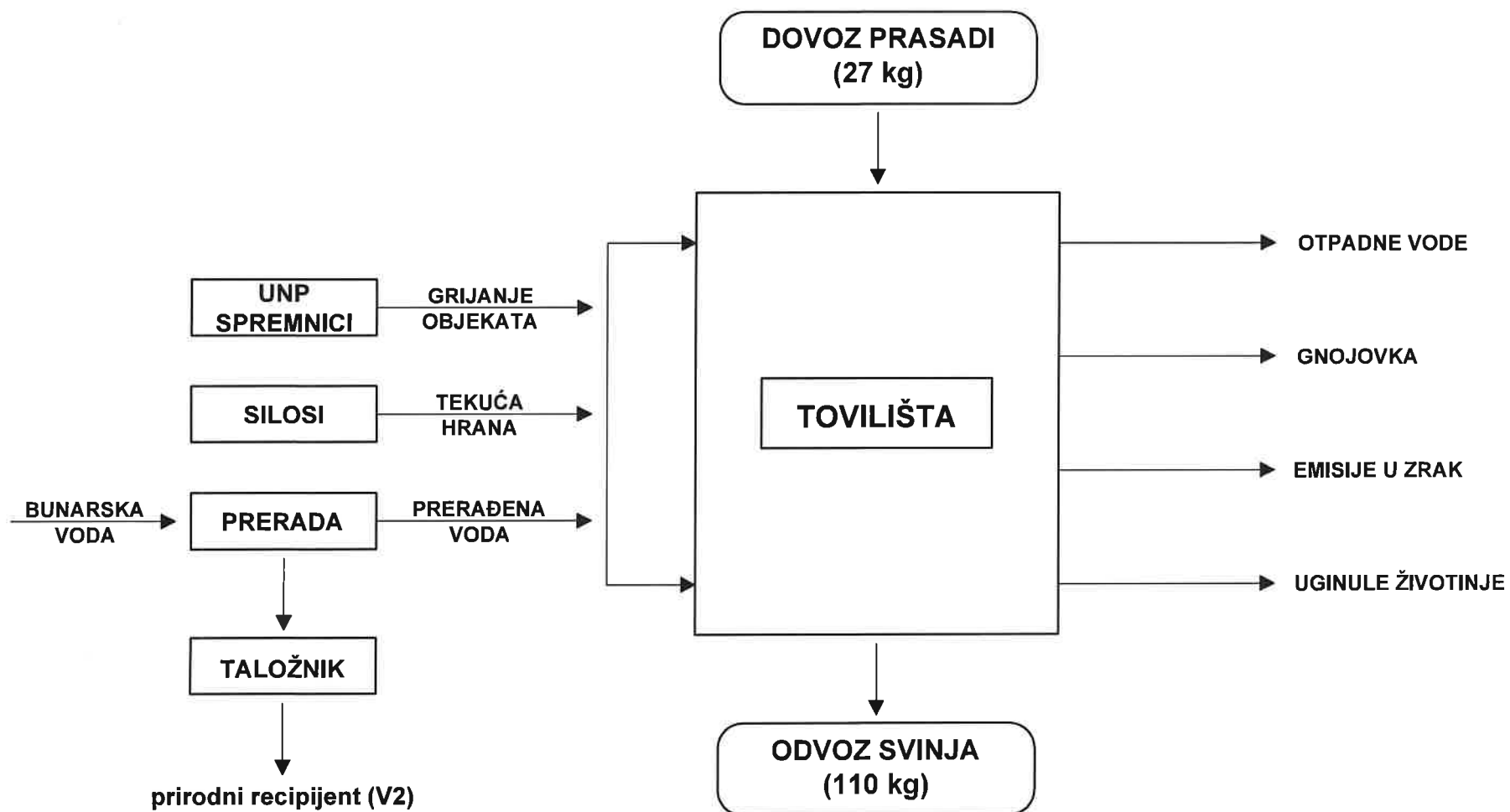
Prilog 2. Blok dijagram tehnološkog procesa na Farmi svinja Sokolovac
